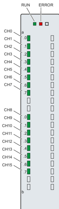
Рисунок 5-1 Светодиодные индикаторы модуля DI 16x24V DC SRC BA
