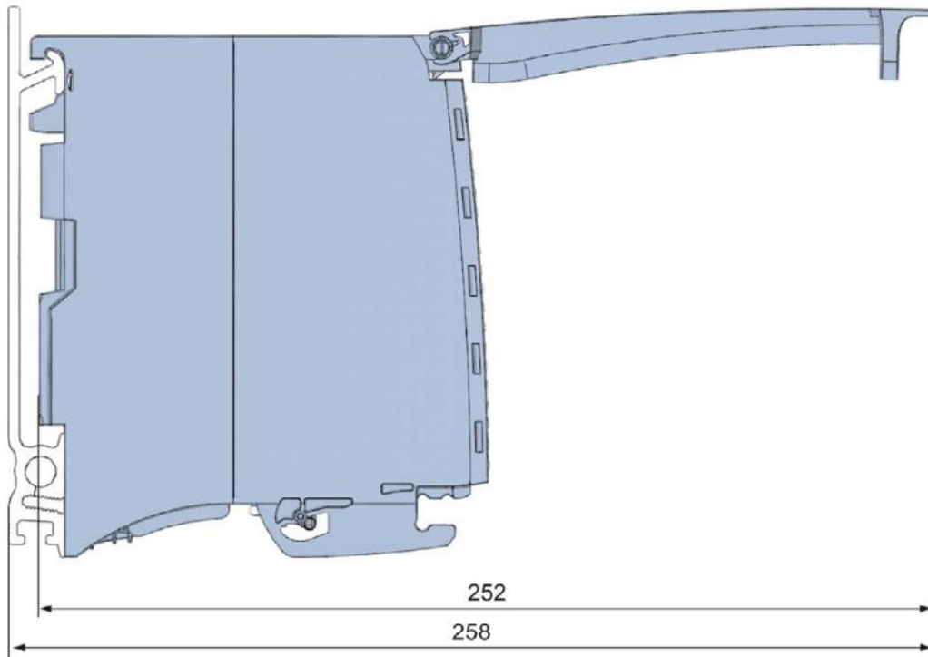
Рисунок А-2 Габаритный чертеж модуля DI 16x24V DC SRC BA вид сбоку, с открытой передней крышкой
