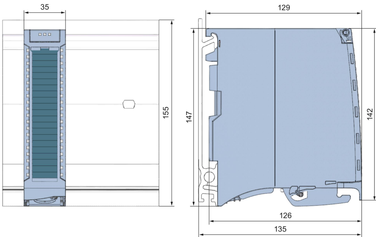
Рисунок А-1 Габаритный чертеж модуля DI 16x24V DC SRC BA
