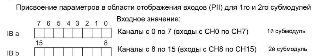
Рисунок 4-2 Пространство адресов для конфигурации модуля в режиме 2х канального входа DI 16x24V DC SRC BA S
