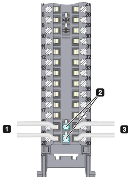
Рисунок 3 -3 Использование перемычек напряжения.
